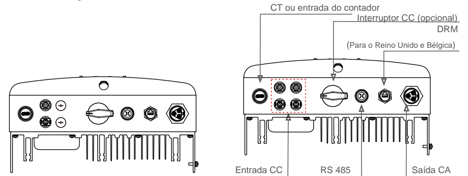
▲ Figura 1.2a Vista lateral inferior (0,7~3,0kW)
