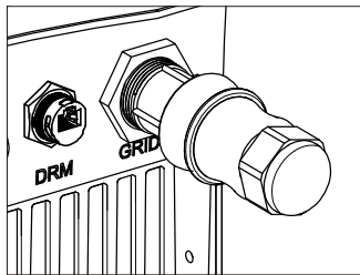
▲ Figura 4.18 Ligue o conector CA ao Inversor
