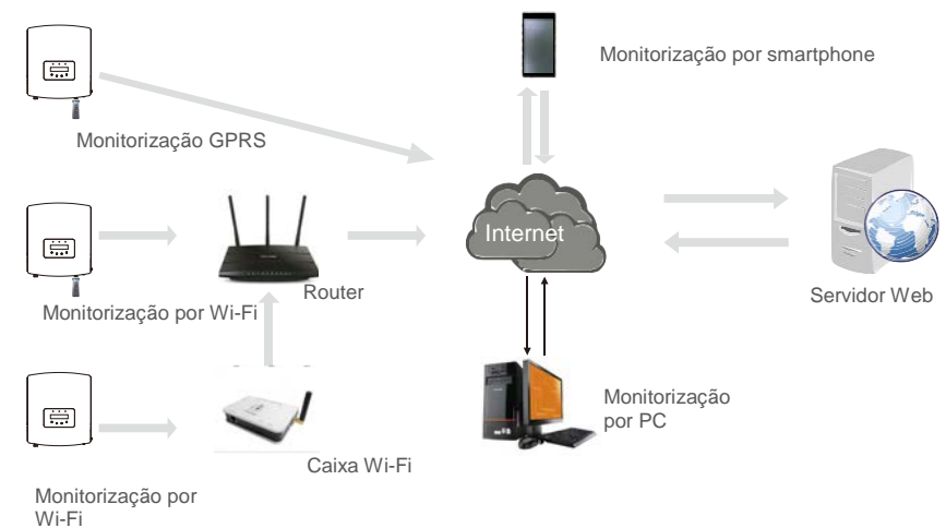
▲ Figura 4.20 Função de comunicação
