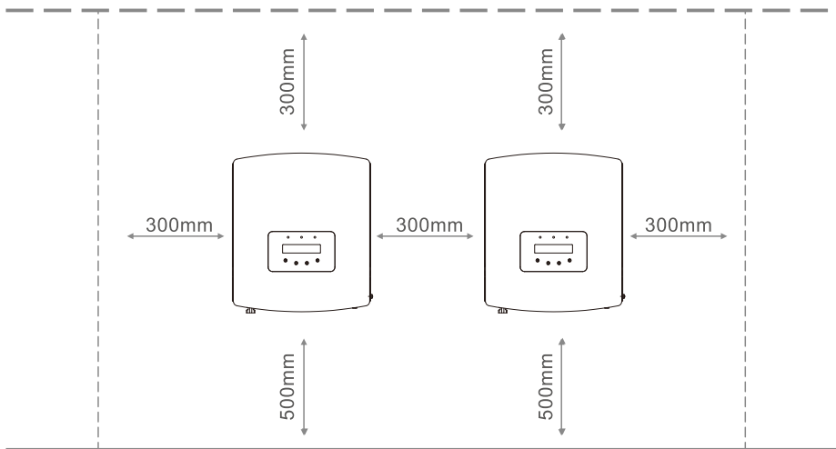
▲ Figura 5.2 Espaço de montagem do inversor
