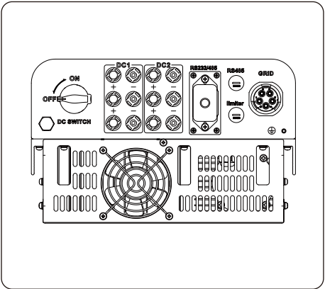
Fig 1.2 Vista Inferior
