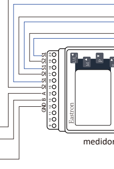
Figura 14 Diagrama da Comunicação do medidor Eastron
