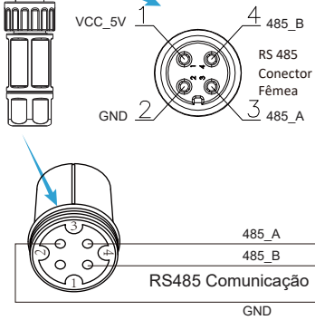
Figura 14 Diagrama da Comunicação do medidor Eastron
