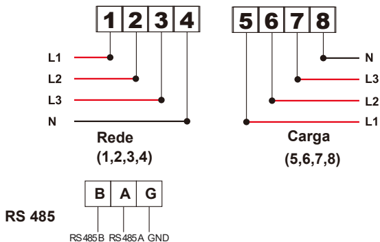
Figura 7.11 Medidor Eastron
