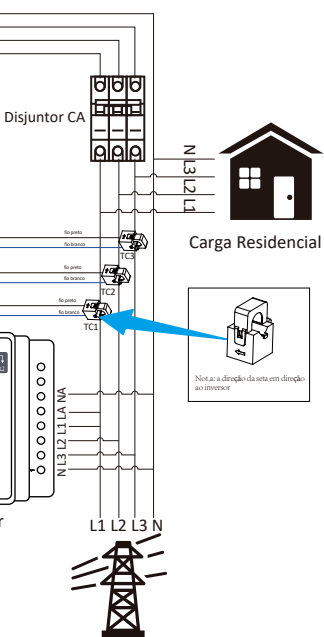
Figura 14 Diagrama da Comunicação do medidor Eastron
