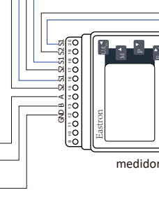
Figura 14 Diagrama da Comunicação do medidor Eastron
