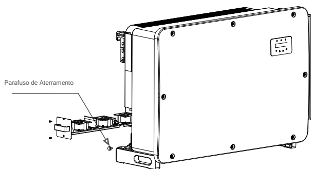
Figura 3.10 Cabo fixo
