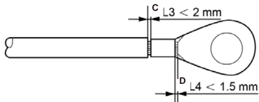
Figura 3.9 Fio decapado
