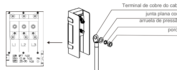
Figura 3.18 Terminal de transferência de alumínio e cobre
