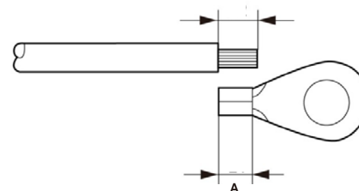
Figura 3.8 Comprimento adequado
