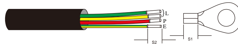
Figura 3.17 Decapar cabo CA
